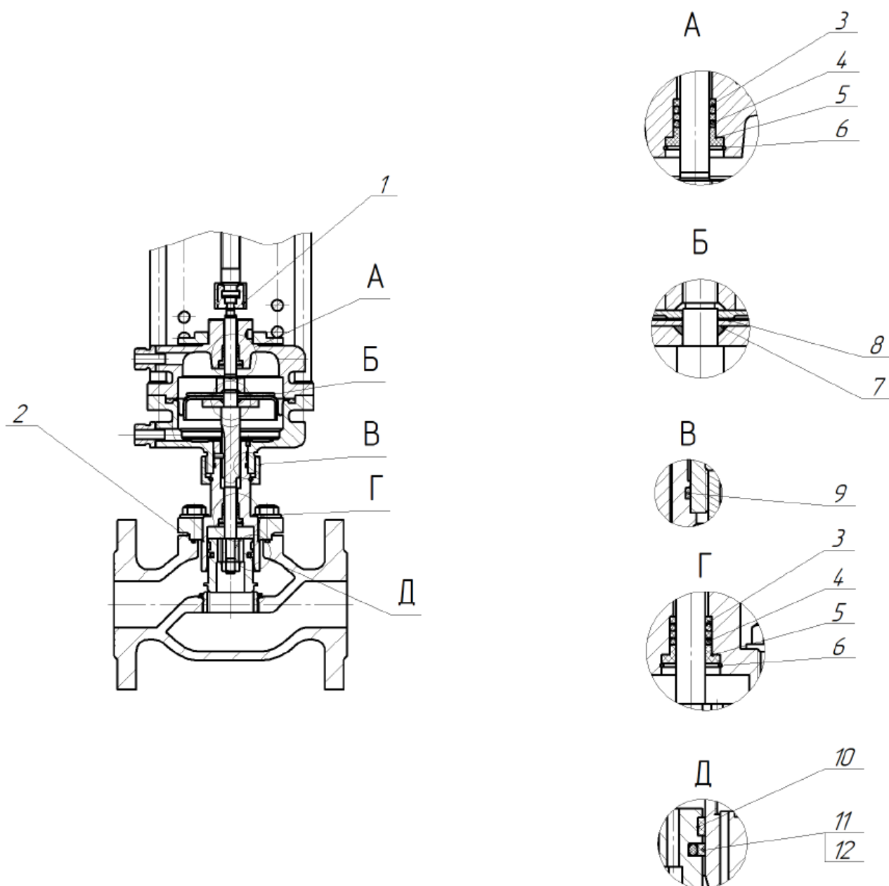
Рис. 5. Ремкомплекты.
