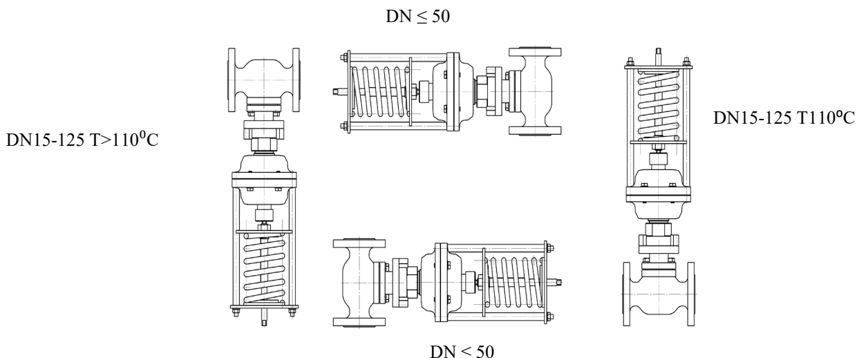
Рис. 3. Схема монтажных положений регулятора перепада давления прямого действия РА-М. Рекомендуемое положение – датчиком вертикально вниз.
