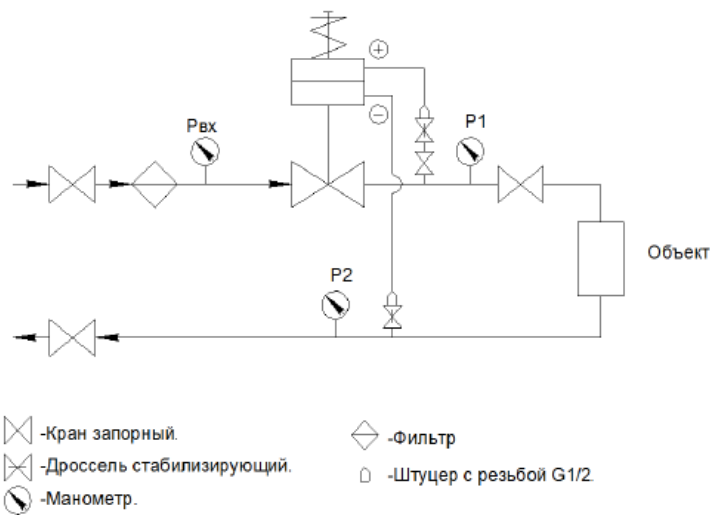
Схема подключения регулятора перепада давления при установке на питающем трубопроводе.
