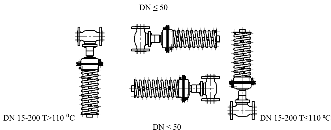
Рис. 3. Схема монтажных положений регулятора давления прямого действия РА-М. Рекомендуемое положение – задатчиком вертикально вниз
