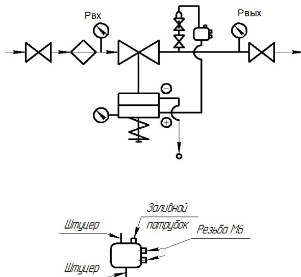
Схема подключения регулятора давления "после себя" РА-А с конденсационно-разделительным сосудом
