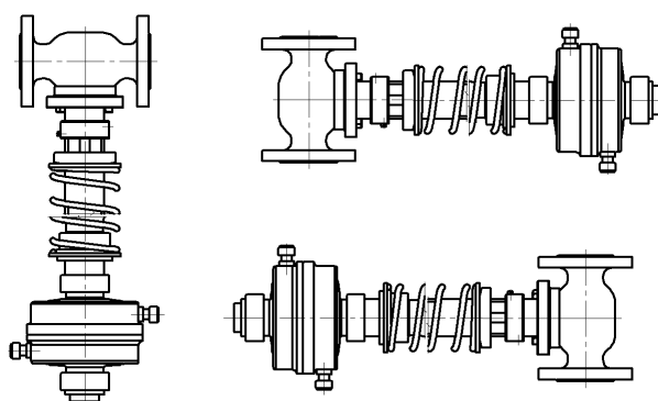
Рис. 3. Схема монтажных положений регулятора давления прямого действия РА-А. Рекомендуемое положение – задатчиком вертикально вниз
